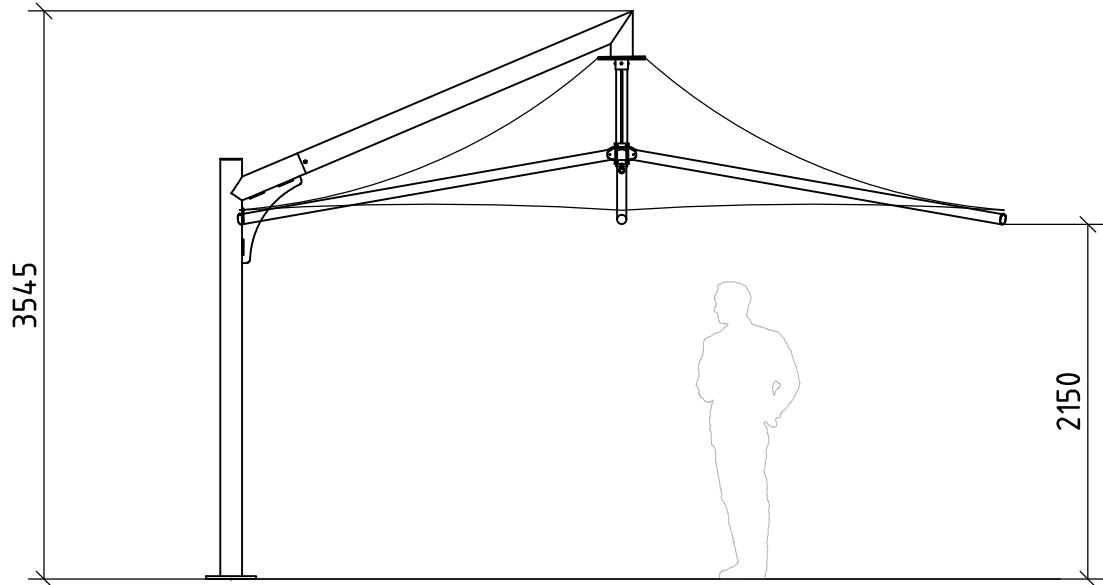
ELEVATION
